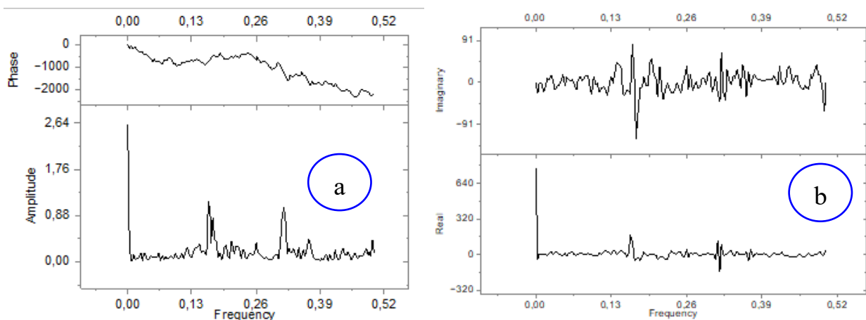
Gambar 7. Perbandingan frekuensi-amplitudo-phase (a) dan frekuensi real-imaginary (b).
