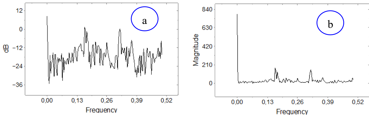
Gambar 8. Perbandingan frekuensi-gelombang suara (a) dan frekuensi-magnitude (b).
