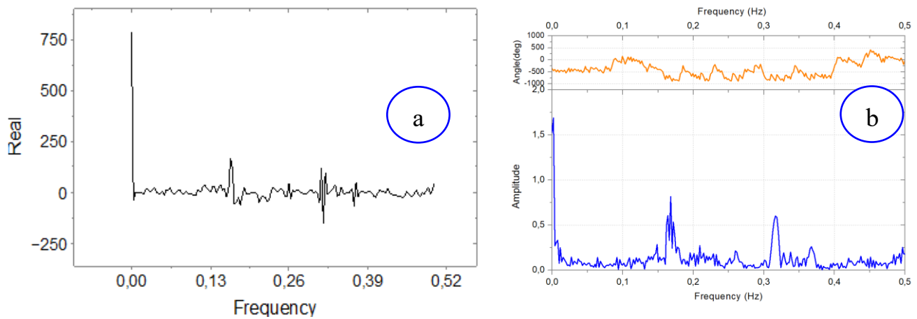
Gambar 10. Perbandingan frekuensi-real (a) dan frekuensi-angel (b).
