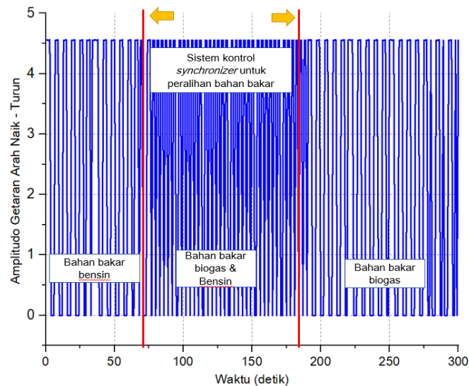
Gambar 6. Data amplitudo getaran dalam sistem digital yang memiliki putaran fast idle .
