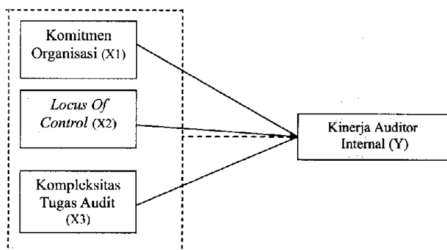
Gambar 1 Kerangka Pikir
