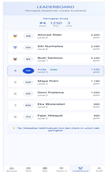
Gambar 9. Rancangan antar muka halaman Leaderboard
